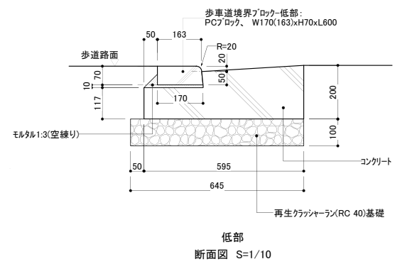
標準・斜部 断面図 S=1/10
