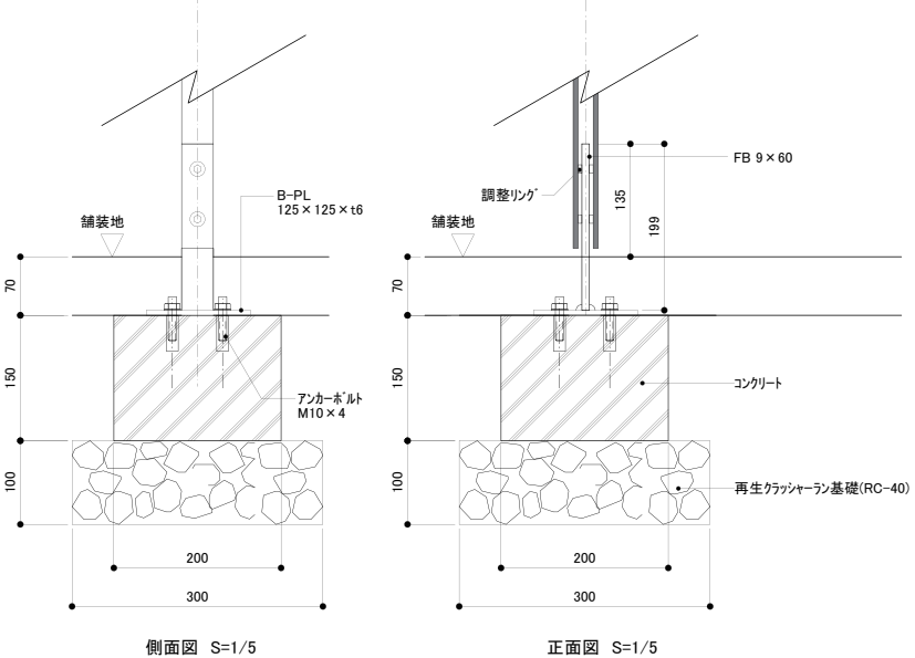
平場部 基礎詳細図(共通)
