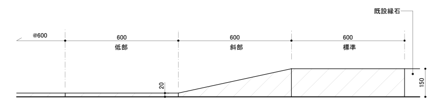
立面図 S=1/10
