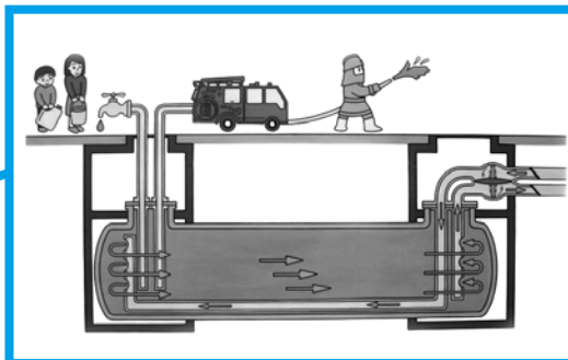
八條小学校の応急給水施設(耐震性貯水槽)
