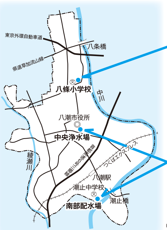
中央浄水場・南部配水場の応急給水施設(災害時給水栓)
