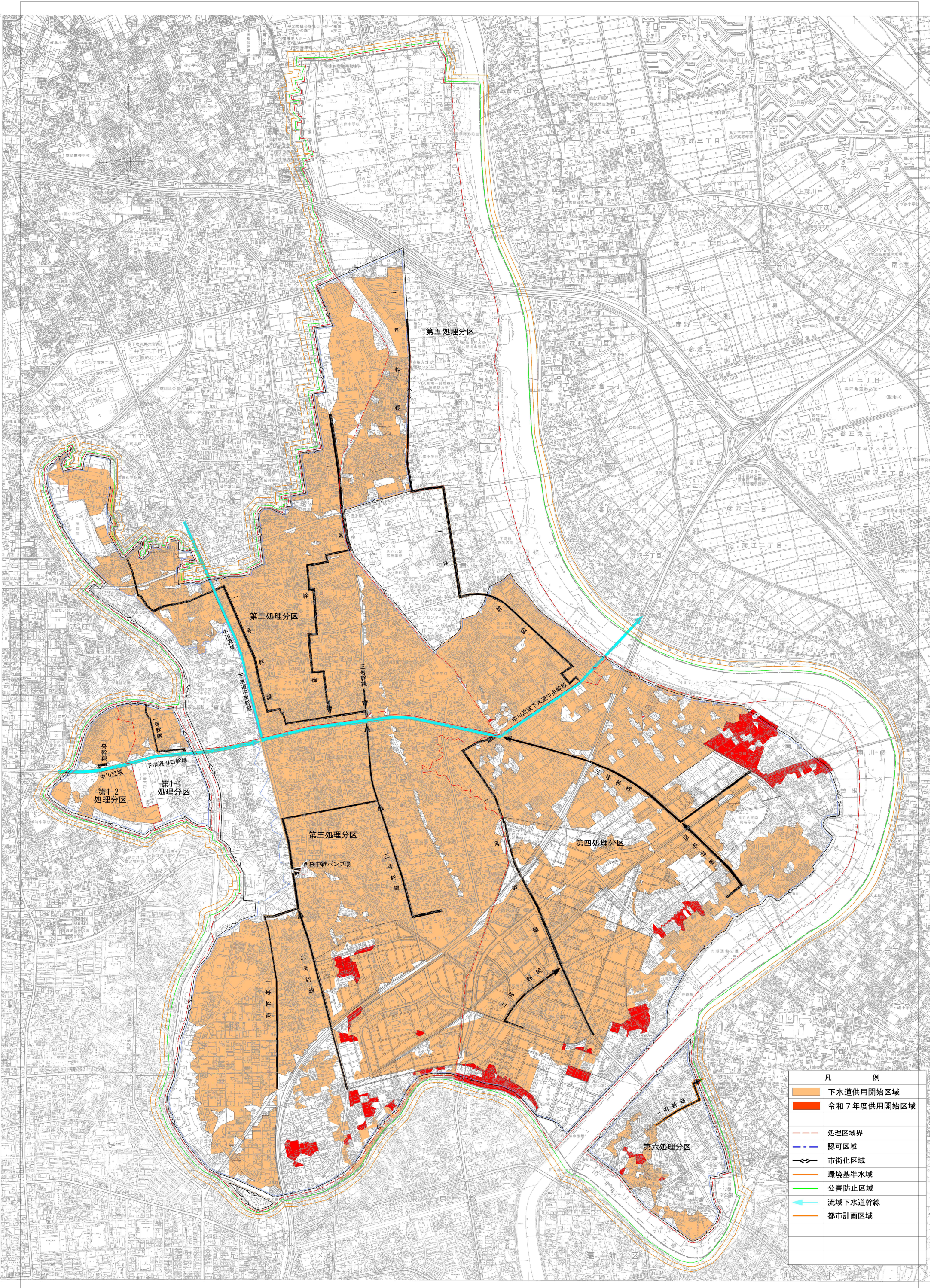
八潮市公共下水道平面図（污水）
