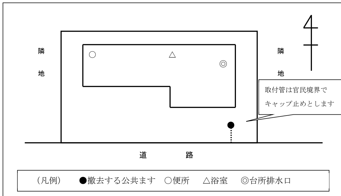
ー公共ます等撤去位置記入例ー
