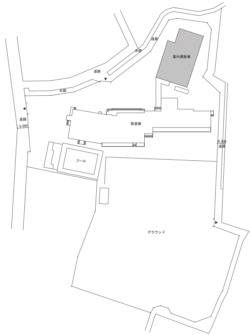
配置図 S=1/600
